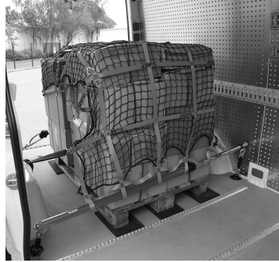
Abb. 16: Verankerung der DoVario-Teleskopstange in den Zurrschienen.
