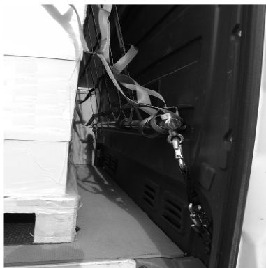
Abb. 6: Die DoVario-Teleskopstange im Einsatz.
