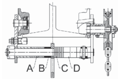
Haspelfahrwerk Do 191/T
