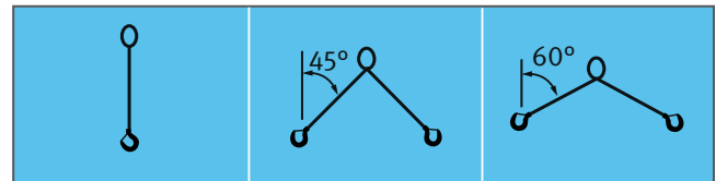
Abb. 2 Beispiele für „Anschlagart direkt“ nach DGUV Information 209-021 „Belastungstabellen für Anschlagmittel aus Rundstahlketten, Stahldrahtseilen, Rundschlingen, Chemiefaserhebebandern, Chemiefaserseilen, Naturfaserseilen“ (Symbolische Darstellung)
