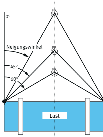
Abb. 5 Neigungswinkel
