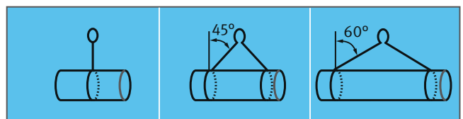
Abb. 3 Beispiele für Anschlagart Schnürgang nach DGUV Information 209-021 „Belastungstabellen für Anschlagmittel aus Rundstahlketten, Stahldrahtseilen, Rundschlingen, Chemiefaserhebebandern, Chemiefaserseilen, Naturfaserseilen“ (Symbolische Darstellung)
