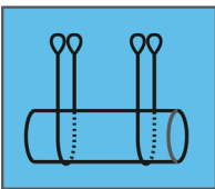
Abb. 4 Beispiel für Anschlagart Hängengang nach DGUV Information 209-021 „Belastungstabellen für Anschlagmittel aus Rundstahlketten, Stahldrahtseilen, Rundschlingen, Chemiefaserhebeebändern, Chemiefaserseilen, Naturfaserseilen“ (Symbolische Darstellung)
